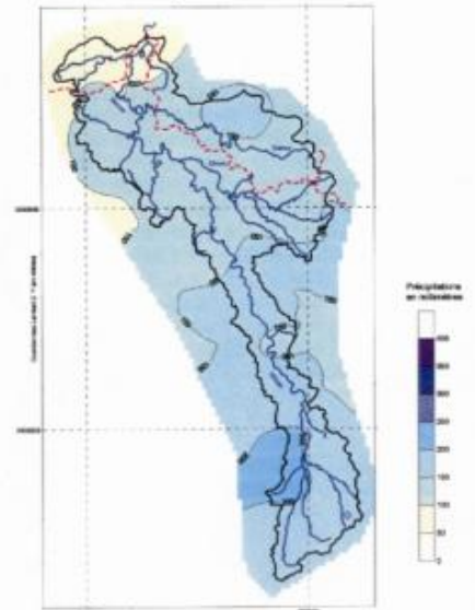
Précipitations sur le bassin-versant de la Meuse, du 4 au 28 avril 83.
